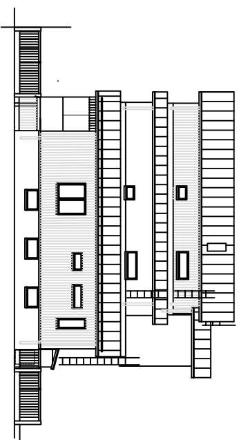
JULKISIVU TORIKADULE KAARKOON
