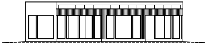
JULKISIVU LOUNAASEEN
