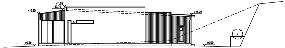
JULKISIVU KAARKKON
